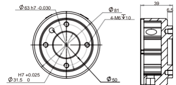
JAKA Zu ® 5 base / flange
