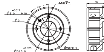
JAKA Zu ® 12 base / flange
